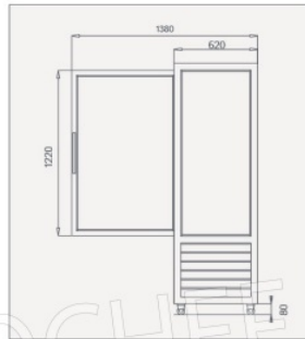
VISTA LATERALE Side view / Seitenansicht / Vue latérale
