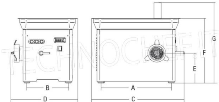
Dimensioni mm
